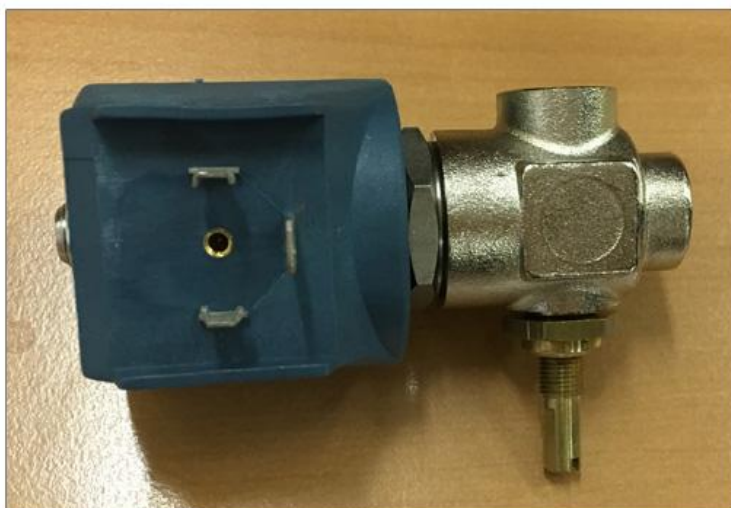
406 Клапан с регулятором Ceme ESQ 9922 Teflon 1/4 "F F (для гладильных столов)
