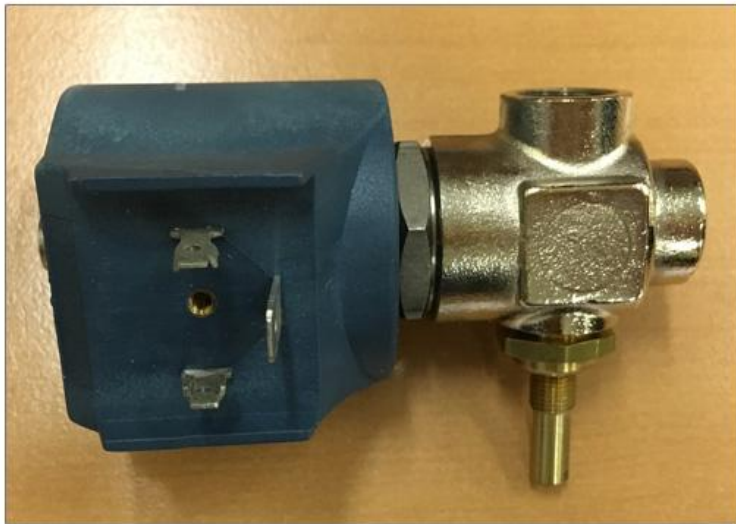
405.24 Клапан Семе ESQ 9922 1/4 "FF (для гладильных столов)
