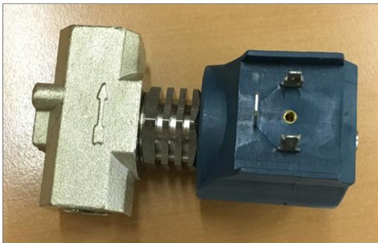
415.A Клапан для гладильных столов Семе ESV 9013 Teflon 3/8 "FF
