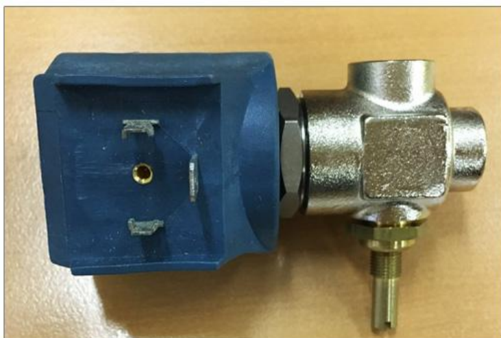
405 Клапан Ceme ESQ 9922 1/4 "F F (для гладильных столов)
